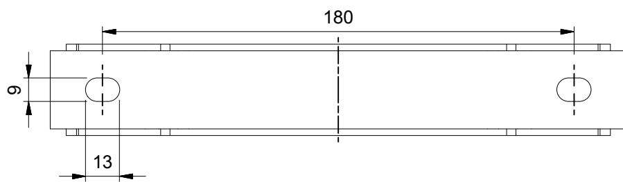
A-A ( 1 : 2 )
