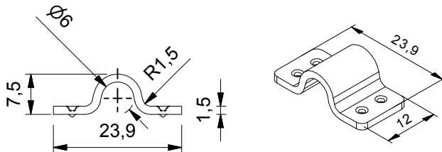
Bridge ( 1 : 1 )
