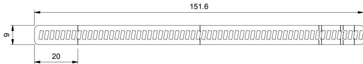
Flat pattern ( 1 : 1 )
