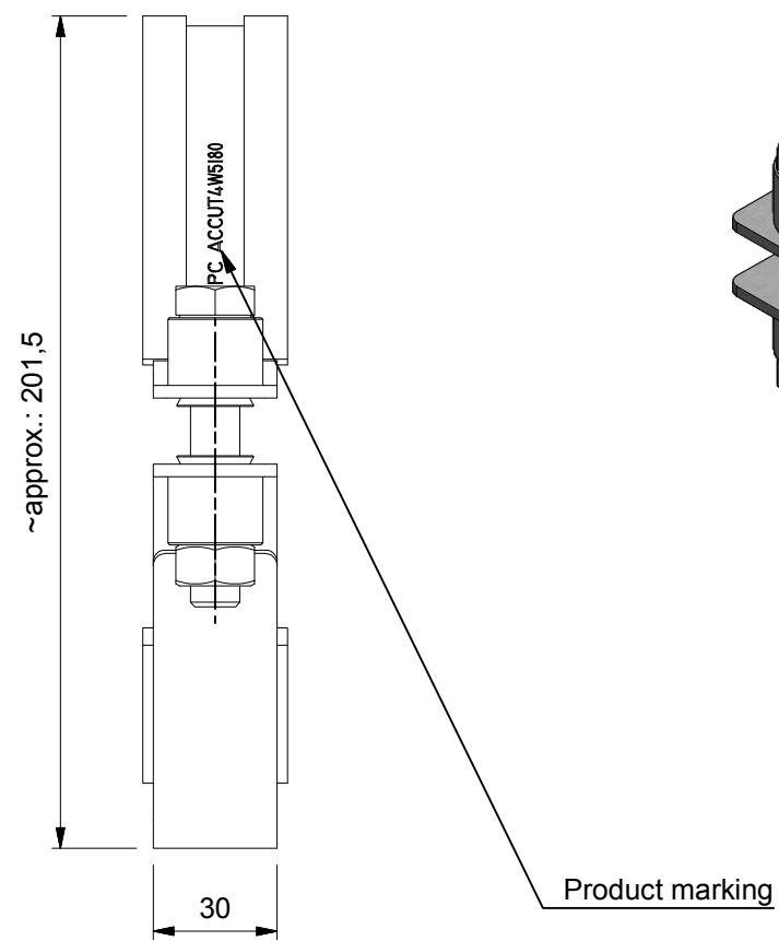
VIEW3 ( 1 : 2 )
